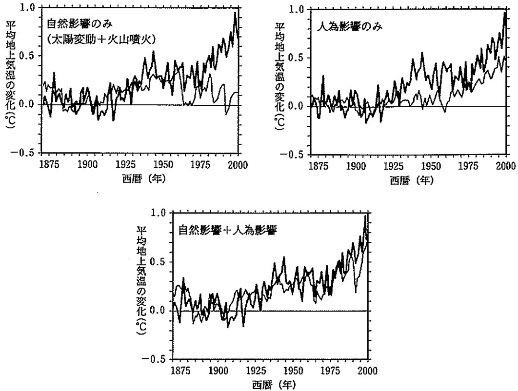
図 V-6 20世紀の気温変化を説明する気候変動モデル 日本第四紀学会編 (2007) 太線は実測値、細線はモデルによる計算値を示す。 各図とも、縦軸の気温は、1881~1990年の平均気温との差を示す。
